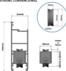
ROLDANA EUROSHOW STRONG CONVENCIONAL
