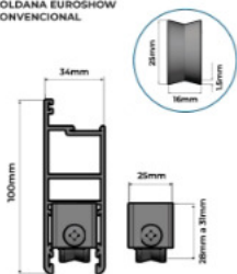
ROLDANA EUROSHOW CONVENCIONAL
