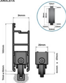
ROLDANA EUROSHOW CANALETA
