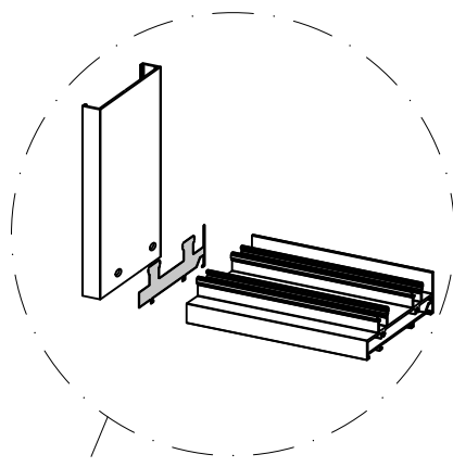
Junta de vedação dos trilhos
