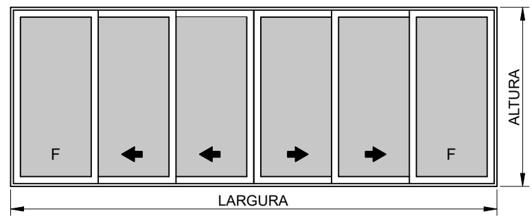
ELEVAÇÃO VISTA EXTERNA SEM ESCALA
