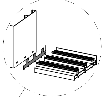
Aplicação da junta de vedação
