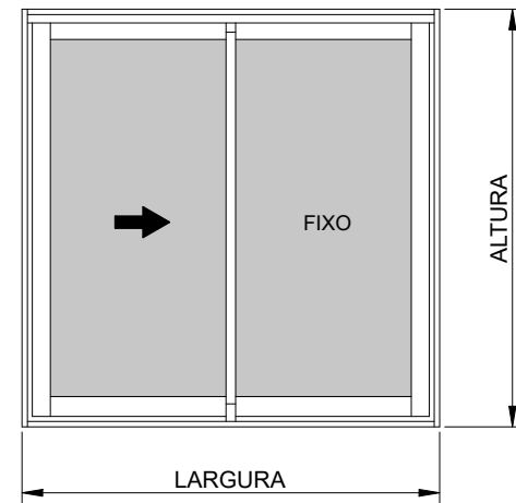
ELEVAÇÃO VISTA EXTERNA SEM ESCALA
