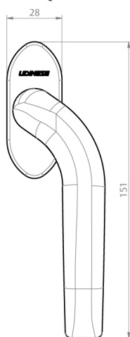
MAÇANETA EXCÊNTRICA ESQUERDA
